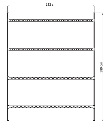
ELEVACIÓN FRONTAL
