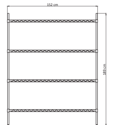
ELEVACIÓN FRONTAL
