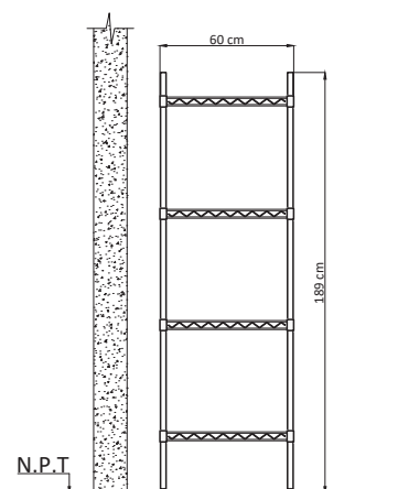
ELEVACIÓN LATERAL
