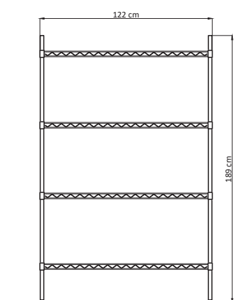
ELEVACIÓN FRONTAL
