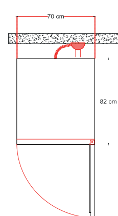
Vista Planta
