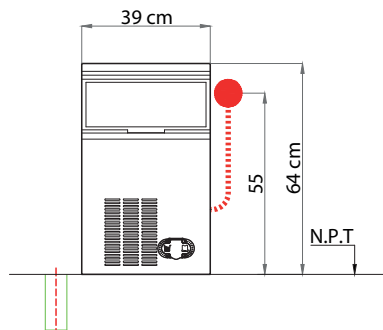
ELEVACIÓN FRONTAL
