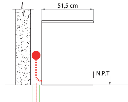
ELEVACIÓN LATERAL
