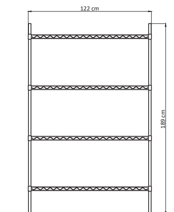
ELEVACIÓN FRONTAL
