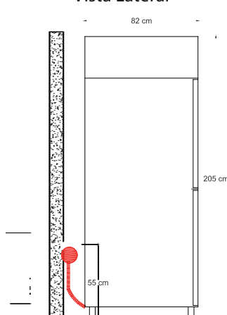
Vista Lateral
