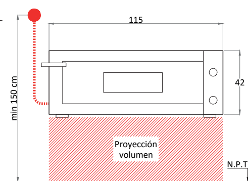
ELEVACIÓN FRONTAL
