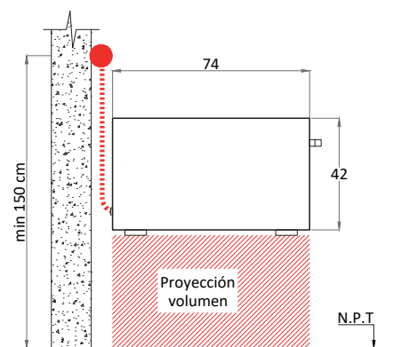
ELEVACIÓN LATERAL
