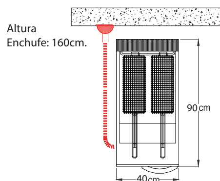
Vista Planta
